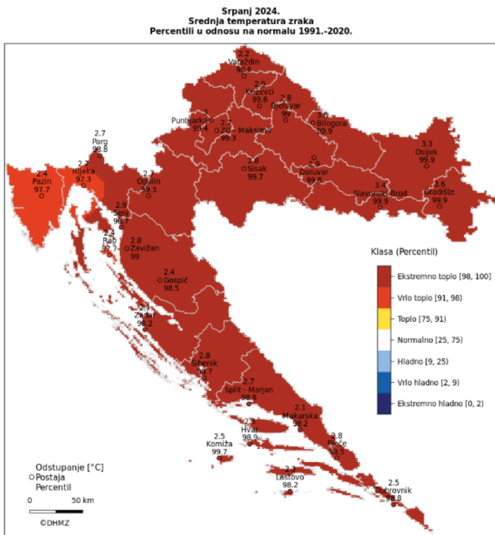
Slika 13. Odstupanje srednje mjesečne temperature zraka za srpanj 2024. godine Izvor: DHMZ
